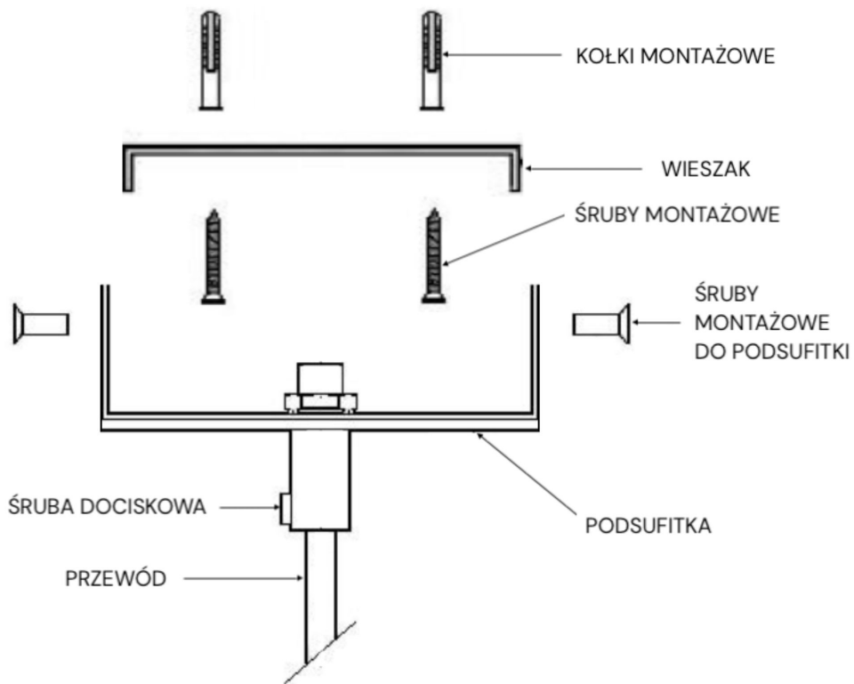
Rys. 1. Montaż oprawy oświetleniowej do sufitu
