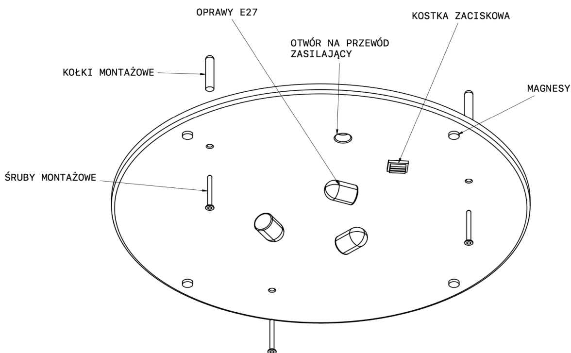
Rys. 1. Montaż oprawy oświetleniowej na przykładzie montażu do sufitu.
