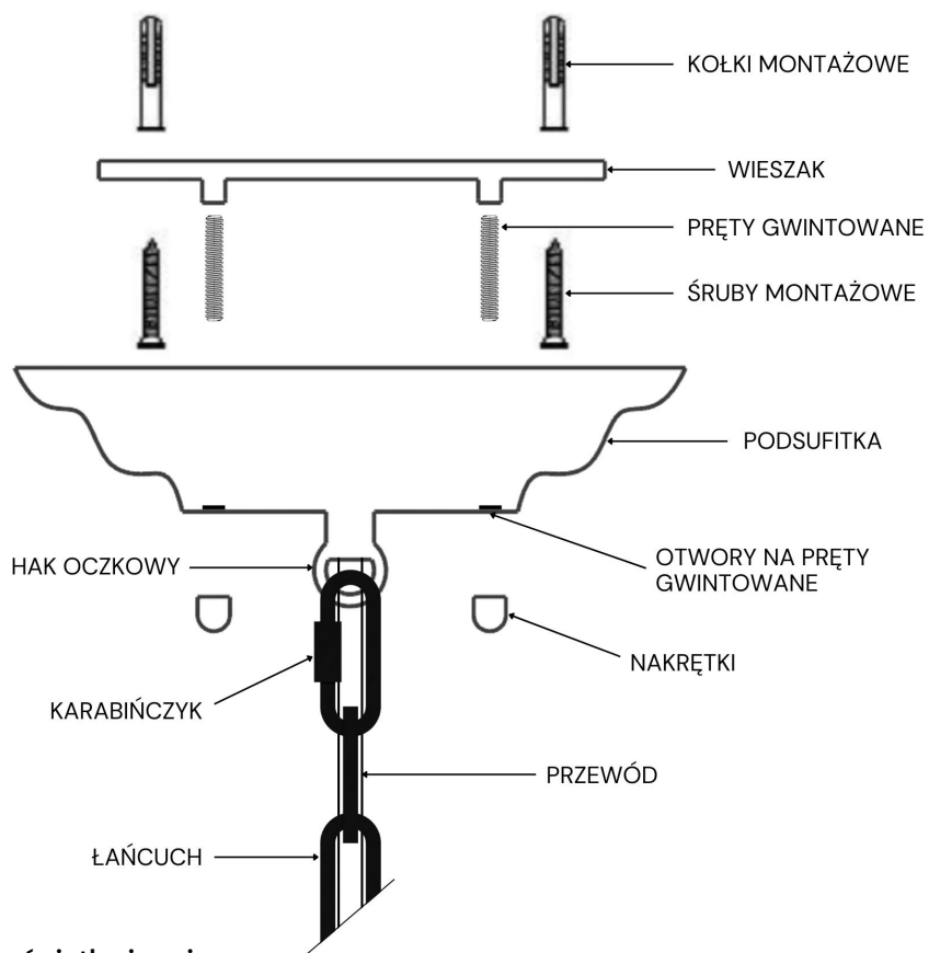
Rys. 1. Montaż oprawy oświetleniowej do sufitu
