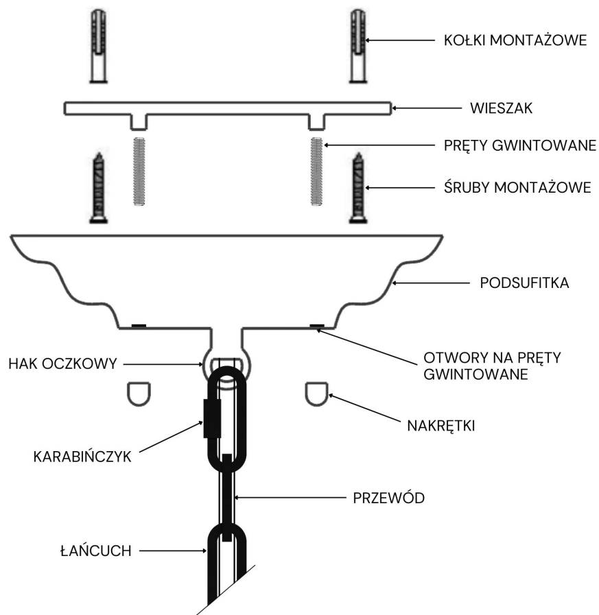
Rys. 1. Montaż oprawy oświetleniowej do sufitu
