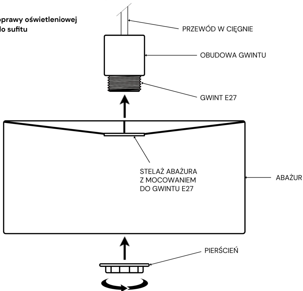
Rys. 2. Montaż abażura do oprawy oświetleniowej
